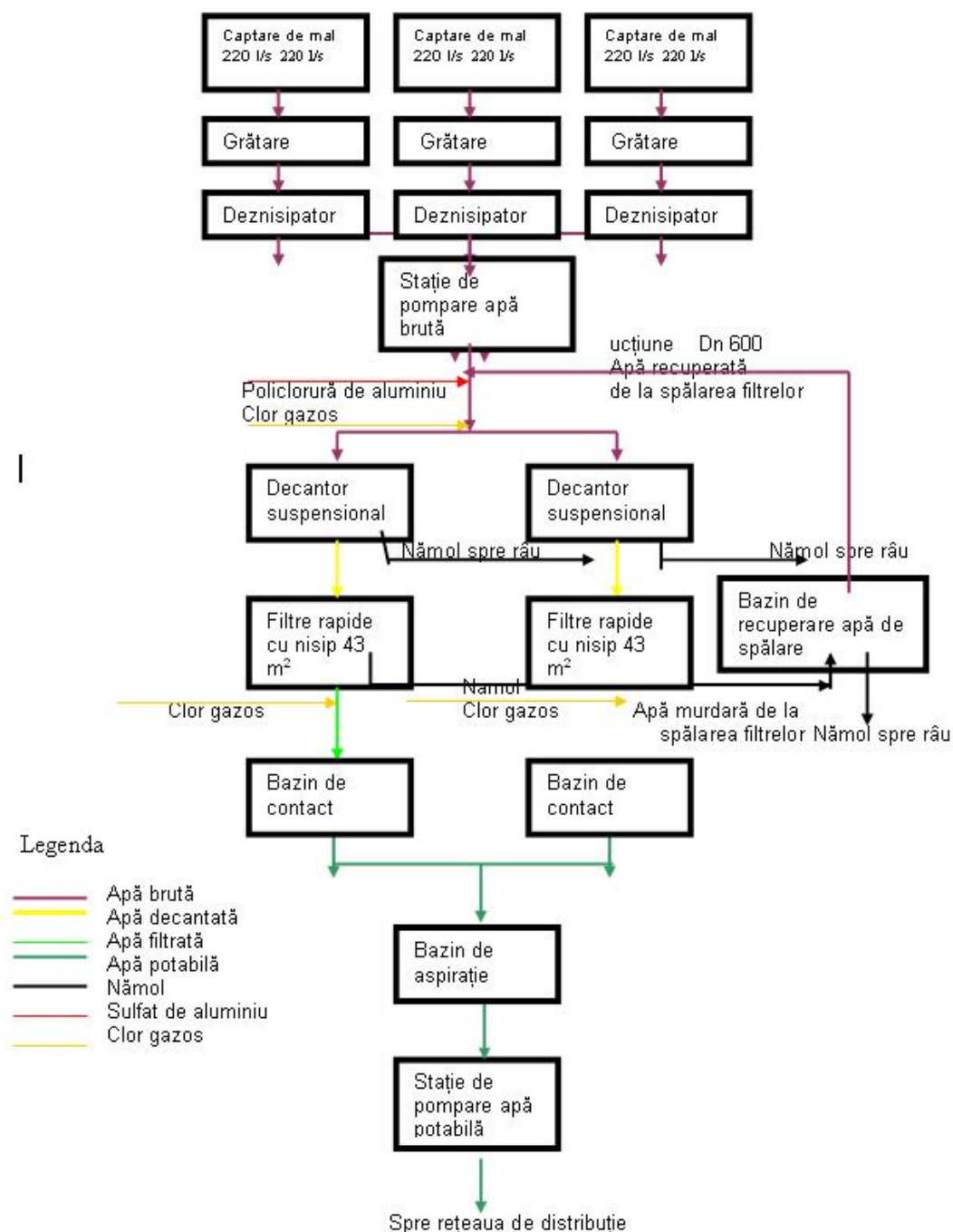
Figura Nr. 2-10 – Stația de tratare a apei Târnăveni – Schemă tehnologică
