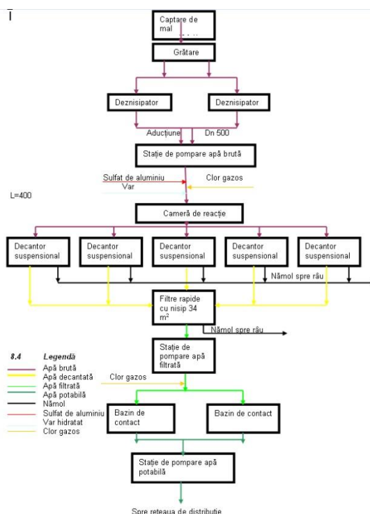
Schema Stației de tratare apă
