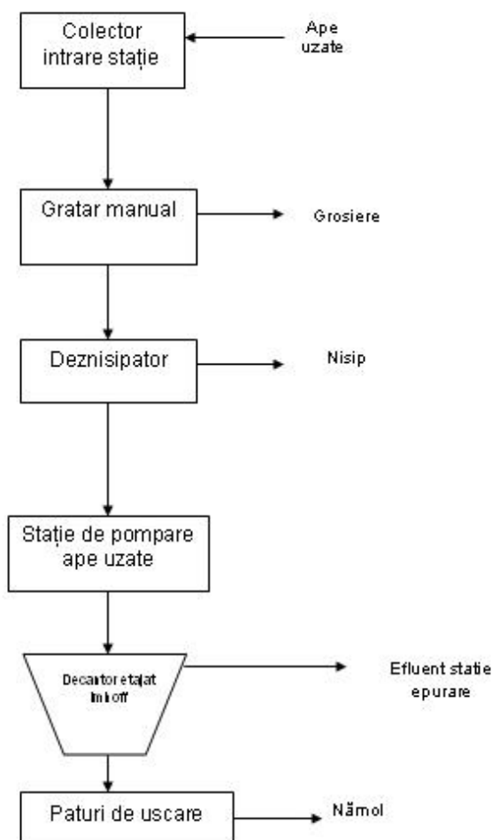
Figura Nr. 2-20 – Schema de tratare a apelor reziduale
